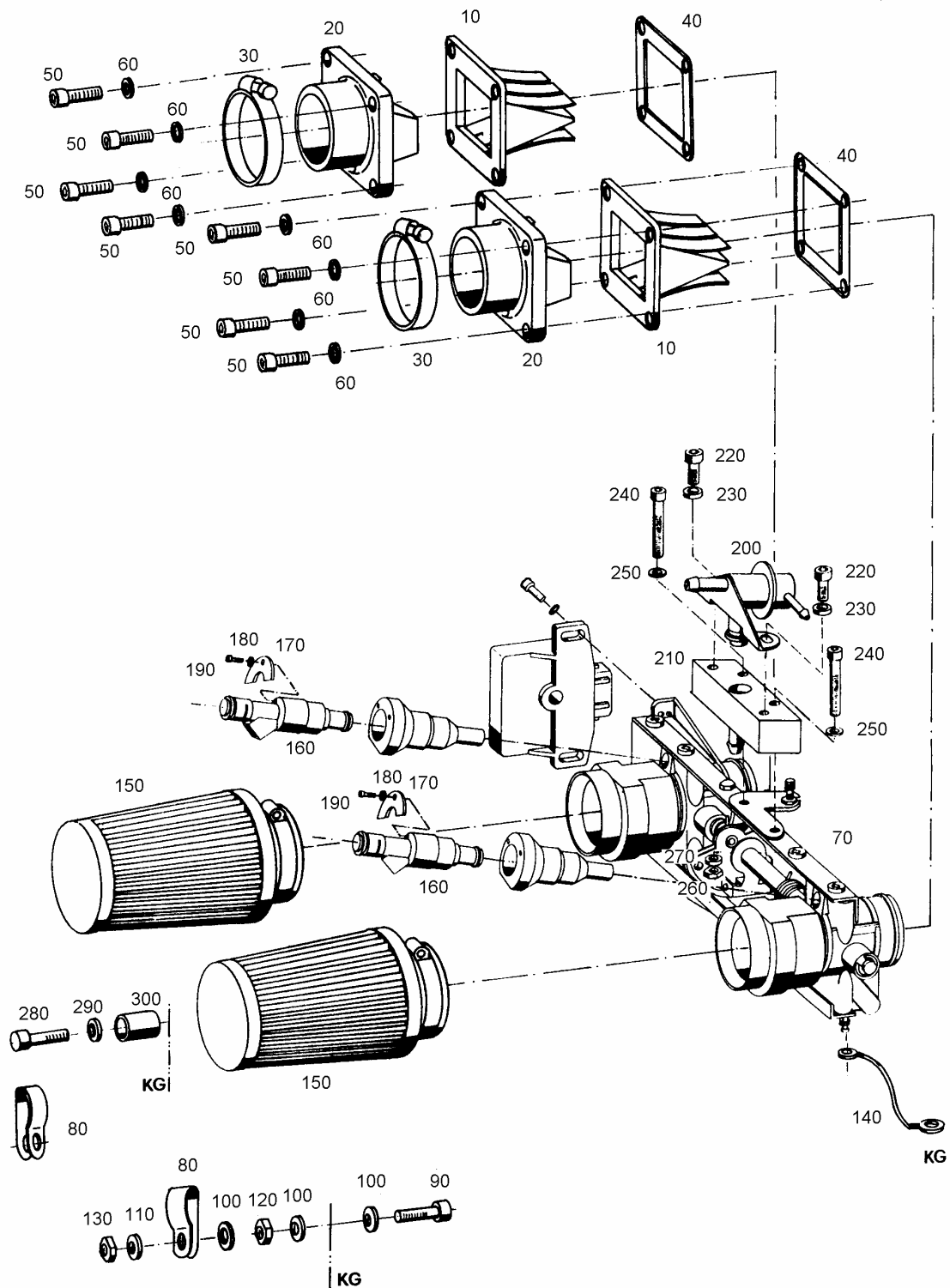
Gemischbildung / Fuel mixture 3202/03 (327 EA)
