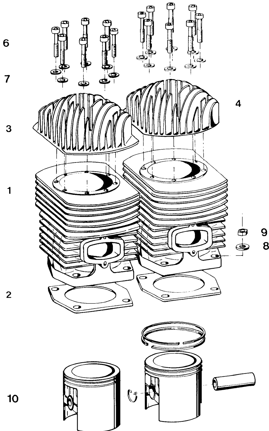
Zylinder Einfachzündung 3202/03 (322H / 322E) Cylinder single ignition
