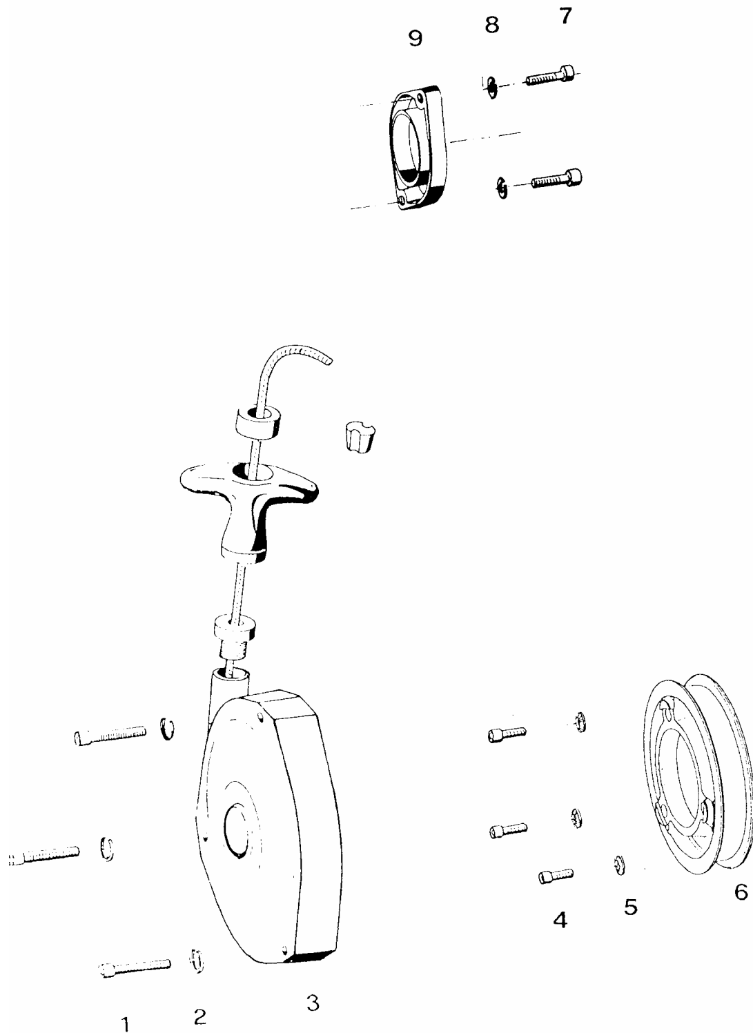
Anwerfvorrichtung / Starting device 3202/03 (275 Y)
