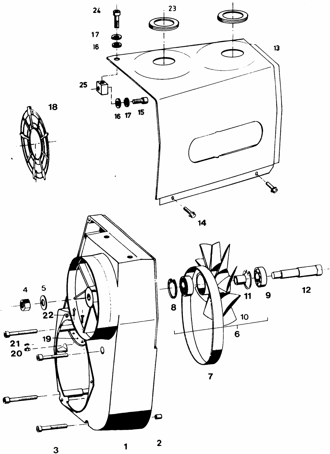
Lüfter Einfachzündung 3202/03 (323G) Fan single ignition
