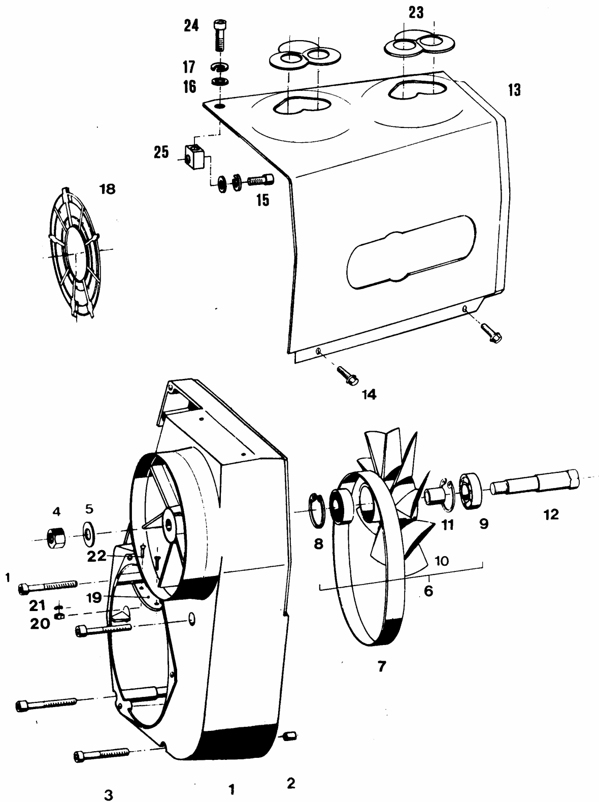
Lüfter Doppelzündung 3202/03 (323 E) Fan dual ignition
